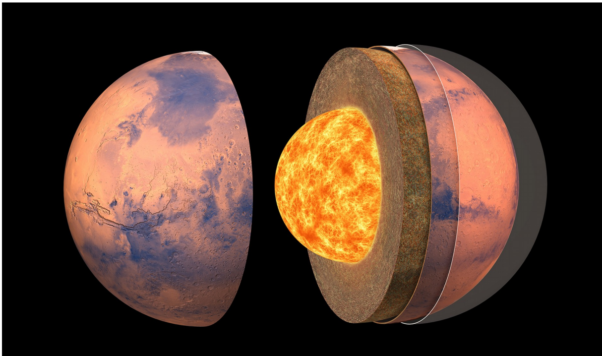
Vue d'artiste de la structure interne de Mars (© IPGP/David Ducros)
